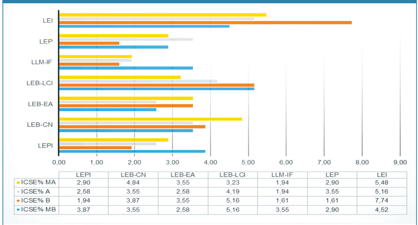
Figura 2. Distribución de los promedios del ICSE en los diferentes programas
