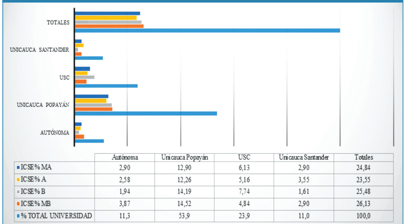
Figura 1. Porcentajes de los resultados del ICSE en Contextos Universitarios
